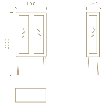
VITRINE
