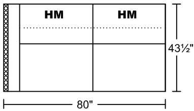
4RA90/LAF 4RAHM/LAF
